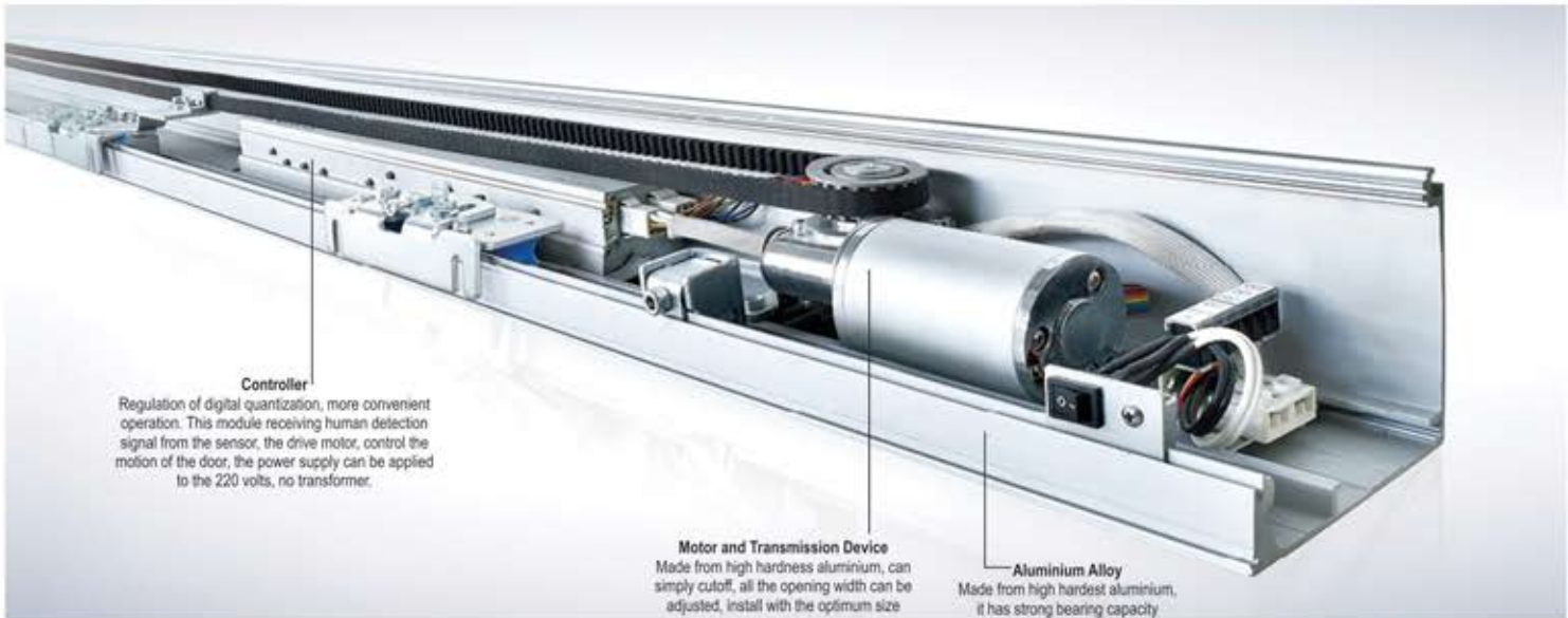
DFASD-22 Automatic Sensor Door
