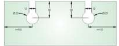
CUTOUT DETAILS OF SSL-44-A1 and SSL-44-A2
