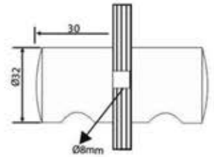
DFDK-1 RG Door Knob
